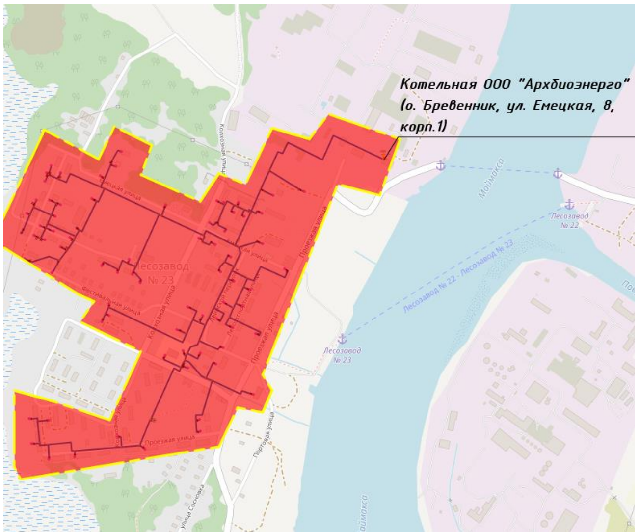
Рисунок 8. Зона действия котельной ООО «Архбиоэнерго» о. Бревенник, ул. Емецкая д. 8, корп.1
