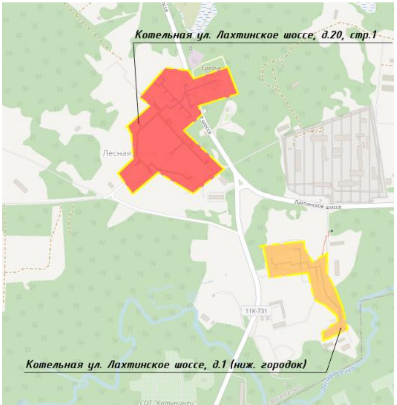
Рисунок 12. Зоны действия котельных ул. Лахтинское шоссе, д. 20, стр. 1 и ул. Лахтинское шоссе, д. 1 (нижний городок)
