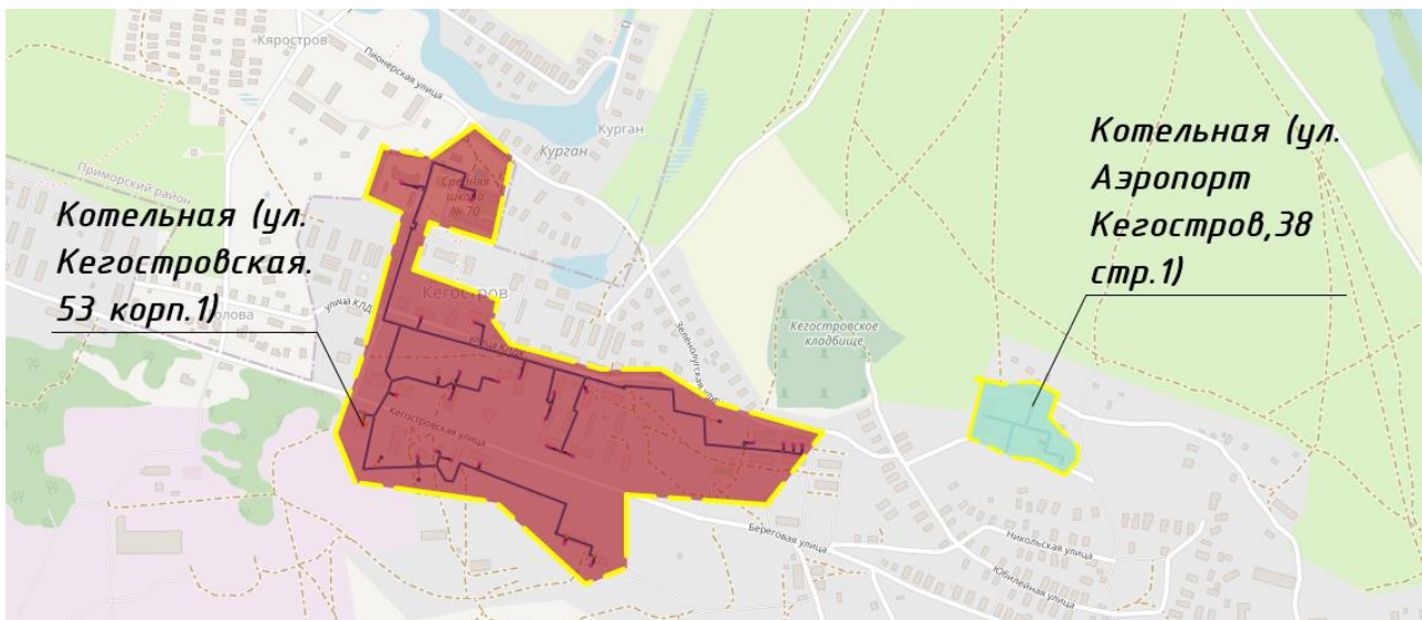
Рисунок 10. Зоны действия котельных ул. Кегаостровская 53, корп. 1 и ул. Аэропорт Кегаостров 38, стр. 1
